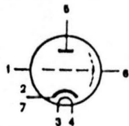
Miniat. B7G
